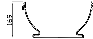
정 면 도 scale : None
