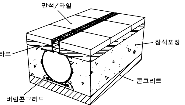
설치예시도 2 scale : None
