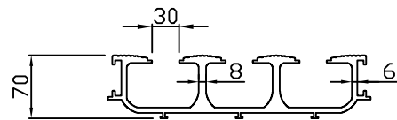
정 면 도 scale : None
